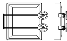
Portella rettangolare orizzontale 420x550 apertura esterna
